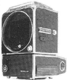
Hasselblad 500 EL/M motorhus Hasselbladsystemets motor-kamera. Kan fjernstyres med radio, timer eller kabel på 120 m. Alle magasiner, objektiver og øvrigt tilbehør passer her til. Kan også bruges til objektiver med automatisk blænde-styring.
